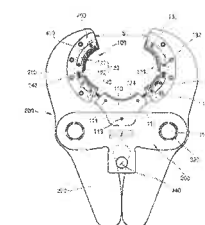
〈파이프 연결용 압착공구 도면〉
